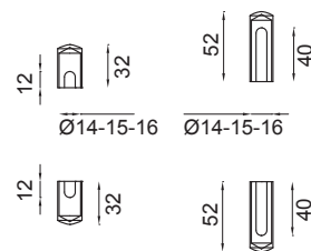
2314/2 set copricerniere lungo con asole lunghe e corte cover hinges set with long or short holes
